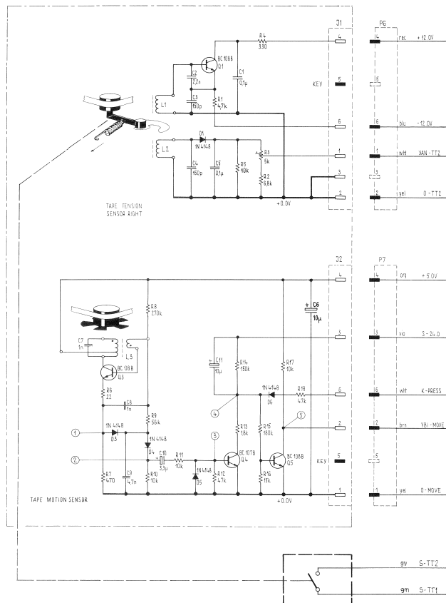
A7 Sensor board, right Abtasterprint, rechts Circuit analyseur, droit 1.067.210
