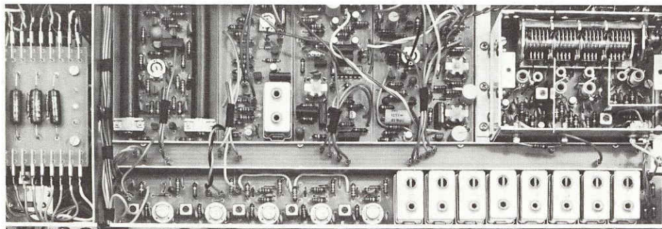
② Hochleistungs-HF-Eingangsteil mit 3 Feldeffekt-Transistoren und 4-fach-Drehkondensator-Abstimmung.
