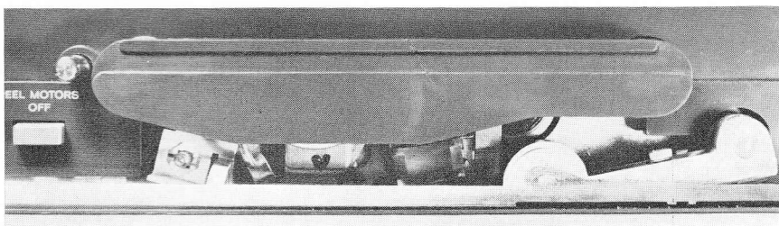
3 Klebeschleife und 45^\circ Schneideschablone an der Kopfabdeckung der REVOX A 77
