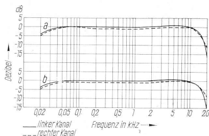
12b Frequenzgang der REVOX A 77 für Aufnahme plus Wiedergabe bei 9,5 cm/s Kurvenpaar a gemessen am Ausgang der Leistungsverstärker Kurvenpaar b gemessen am Ausgang der 8-W-Endstufen
