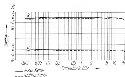
12c Frequenzgang der REVOX A 77 für Aufnahme plus Wiedergabe bei 19 cm/s Kurvenpaar a gemessen am Ausgang der Leistungsverstärker Kurvenpaar b gemessen am Ausgang der 8-W-Endstufen
