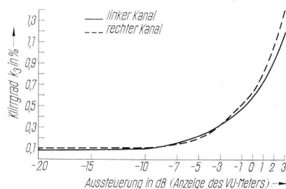
13b Kubischer Klirrgrad ( k_3 ) bei 1 kHz und 9,5 cm/s in Abhängigkeit von der Bandaussteuerung, gemessen am Ausgang der Endverstärker
