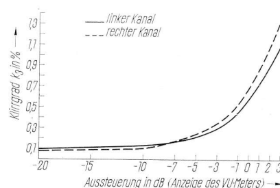
13a Kubischer Klirrgrad ( k_3 ) bei 1 kHz und 9,5 cm/s in Abhängigkeit von der Bandaussteuerung, gemessen am Ausgang der Leistungsverstärker
