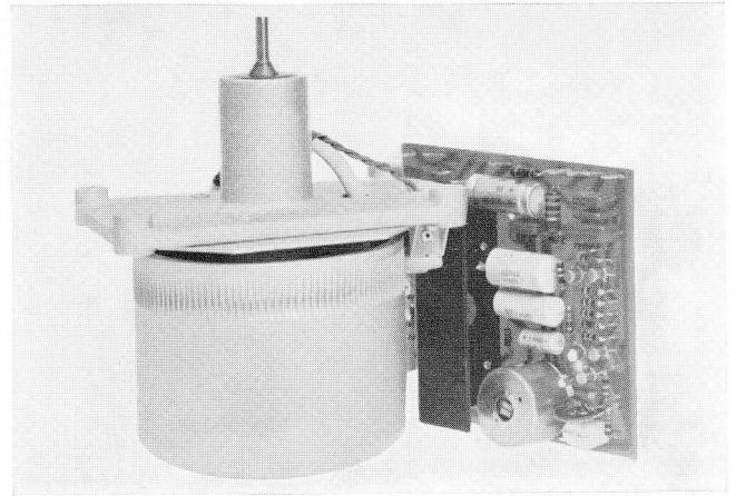
5 Der Tonwellenmotor der A 77 mit der die Steuer- und Regelelektronik enthaltenden Printplatte. (Am oberen Ende des Motorgehäuses sind deutlich die zur Erzeugung der Umlauf-Kontrollfrequenz erforderlichen Einfräsungen, auf der rechten Seite des Motorträgers die hierfür erforderliche Abtastspule sichtbar.)
