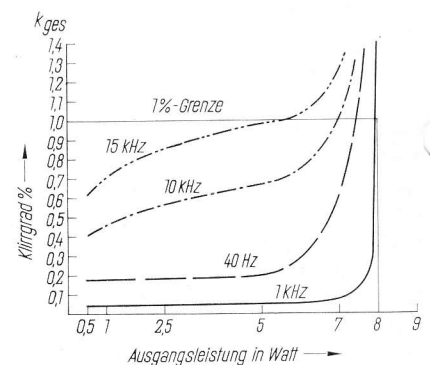
11b Klirrradverlauf ( k_{ges} ) von Leistungs- plus Endverstärker im rechten Kanal der REVOX A 77 an 8 Ohm reell in Abhängigkeit von der Ausgangsleistung für den Frequenzbereich von 40 Hz bis 15 000 Hz
