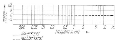
9 Frequenzgang der REVOX A 77 bei Benutzung als Verstärkeranlage (Leistungs- plus Endverstärker).
