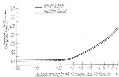
13d Kubischer Klirrgrad ( K_3 ) bei 1 kHz und 19 cm/s in Abhängigkeit von der Bandaussteuerung, gemessen am Ausgang der Endverstärker
