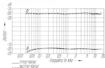
12a Frequenzgang der REVOX A 77 bei der Wiedergabe von Bezugsbändern nach DIN 45513 Kurvenpaar a für 9,5 cm/s Kurvenpaar b für 19,0 cm/s
