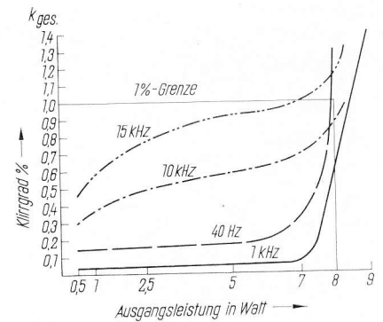
11a Klirrradverlauf ( k_{ges} ) von Leistungs- plus Endverstärker im linken Kanal der REVOX A 77 an 8 Ohm reell in Abhängigkeit von der Ausgangsleistung für den Frequenzbereich von 40 Hz bis 15 000 Hz
