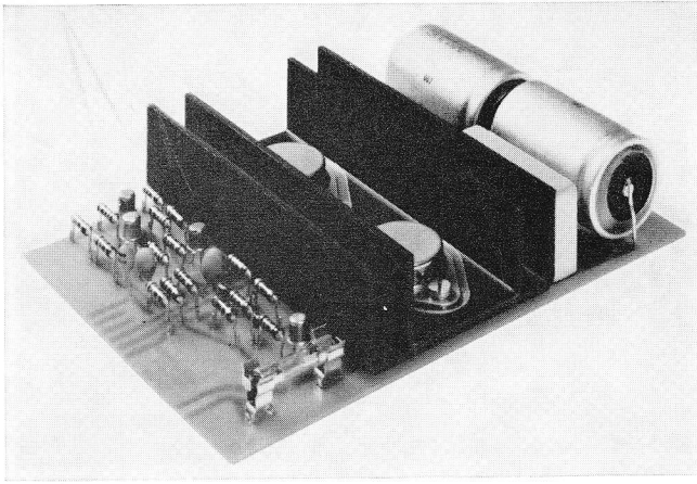
4 Steckbare 8-Watt-Endstufe für die REVOX A 77. (Auf der linken Seite der Steckkarte sind deutlich die Kontaktbahnen erkennbar, die in die Kontaktleisten im Gerätechassis eingreifen.)
