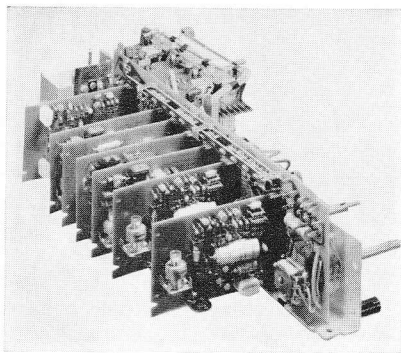
8 Auf einer leicht auszubauenden Platine haben — mit Ausnahme der beiden Endstufen — sämtliche Steckkartenverstärker, die beiden VU-Meter, sowie sämtliche Bedienelemente ihren Platz in der REVOX A 77 gefunden.
