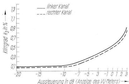
13c Kubischer Klirrgrad ( K_3 ) bei 1 kHz und 19 cm/s in Abhängigkeit von der Bandaussteuerung, gemessen am Ausgang der Leistungsverstärker
