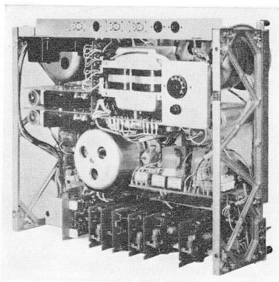
6 Rückansicht der REVOX A 77. (Ein stabiles verwindungssteifes Druckguß-Chassis trägt: oben die Wickelmotore, das stabilisierte Stromversorgungsteil und die beiden einsteckbaren 8-Watt-Endverstärker; in der Mitte den Tonwellenmotor und die Steuerrelais für die Laufwerkfunktionen; unten die steckbaren Aufsprech- und Wiedergabeverstärker, den Oszillator für die Vormagnetisierungs- und Löschfrequenz sowie [im Bild nicht sichtbar] sämtliche Verstärker-, Bedien- und Kontrollelemente.)
